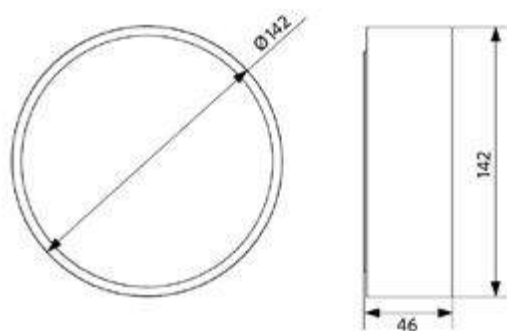
LEDCeilingLu-E Rd142
